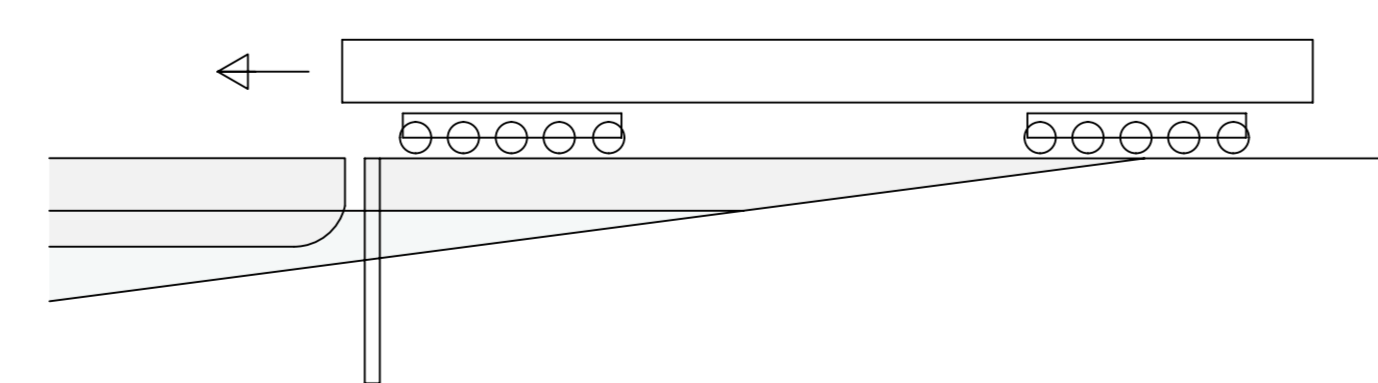
Prinzipschnitt Vorschub auf Pontons
